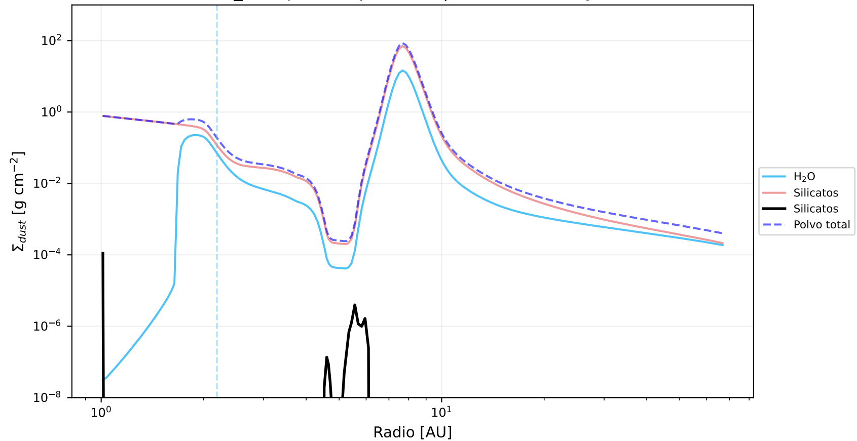
\Sigma_{\text{dust}} por componente | t = 2.88\text{e}+06 yr
